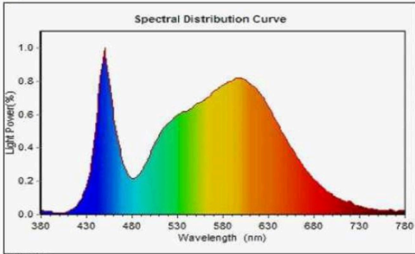
光谱分布
