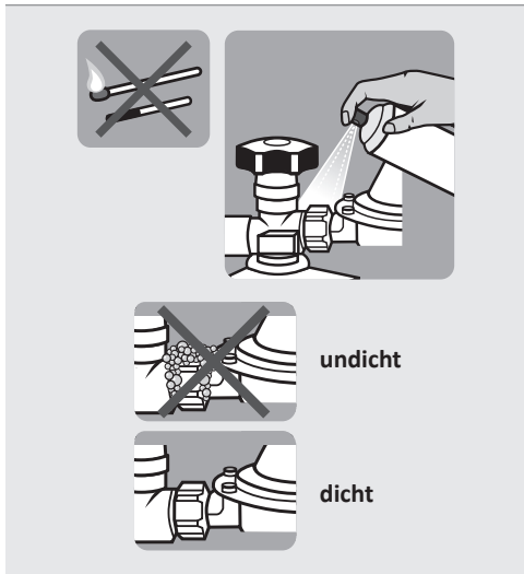
Abb.2: Dichtheitsprüfung
