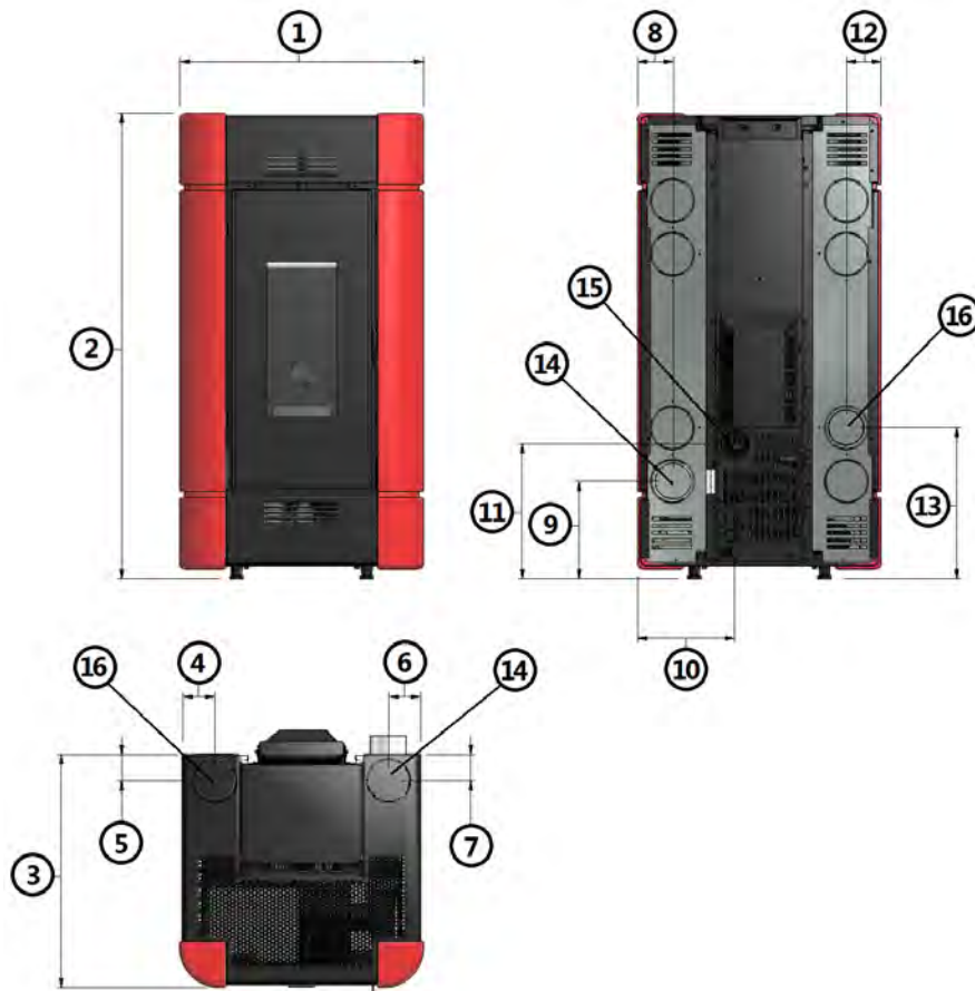
Fig. 16 - Allgemeine Abmessungen: Sire 3 Plus
