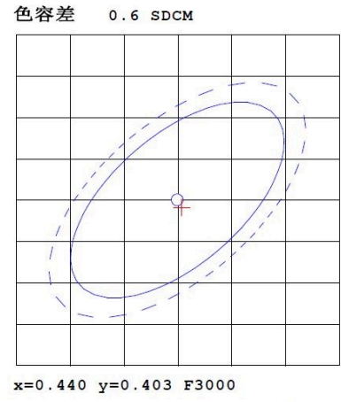
CIE1931色品图
