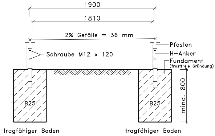
Schnitt A-A
